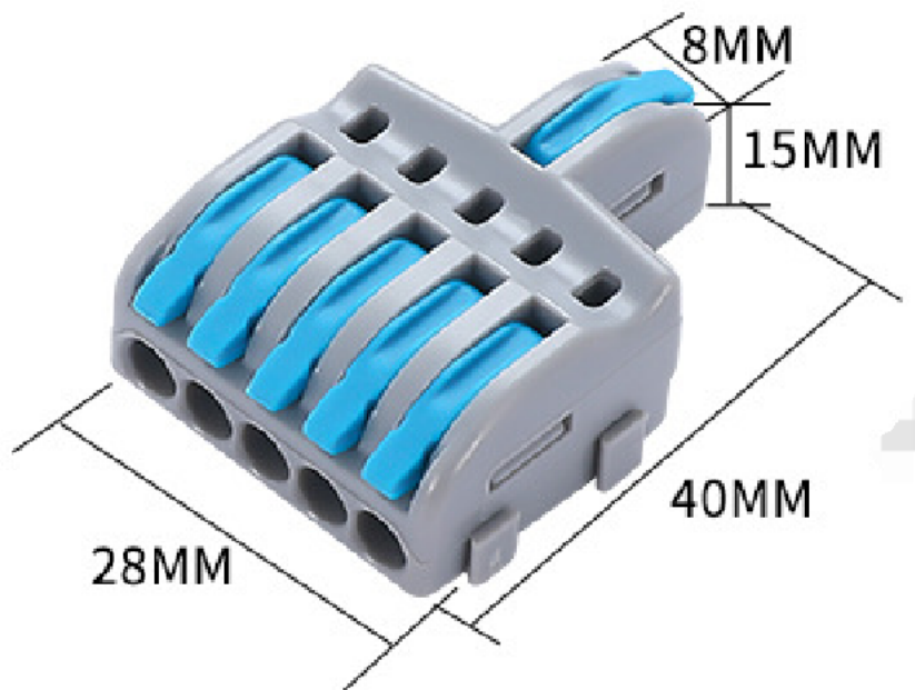
一进五出蓝色接线端子
